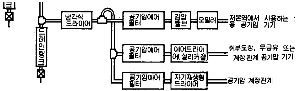
그림 5.4 에어 실린더 구동회로
